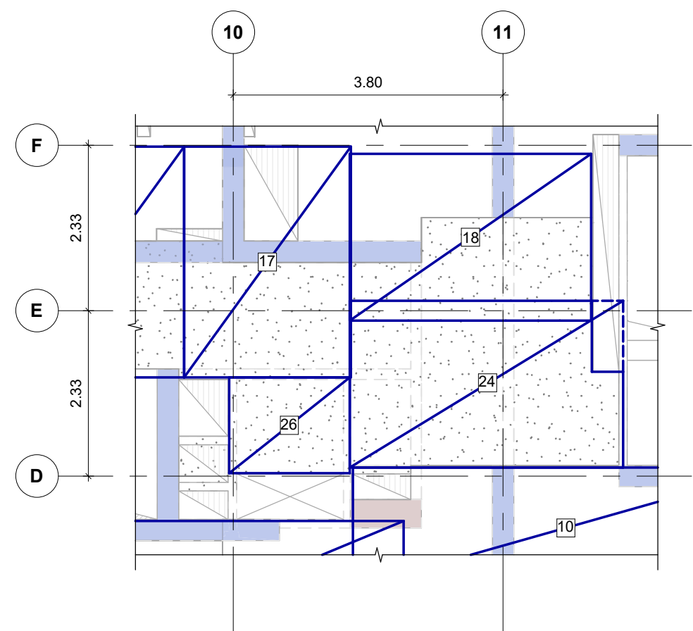
PLANTA DE REFUERZO SUPERIOR PISO 14 Y PISO 15 Escala 1 : 75
