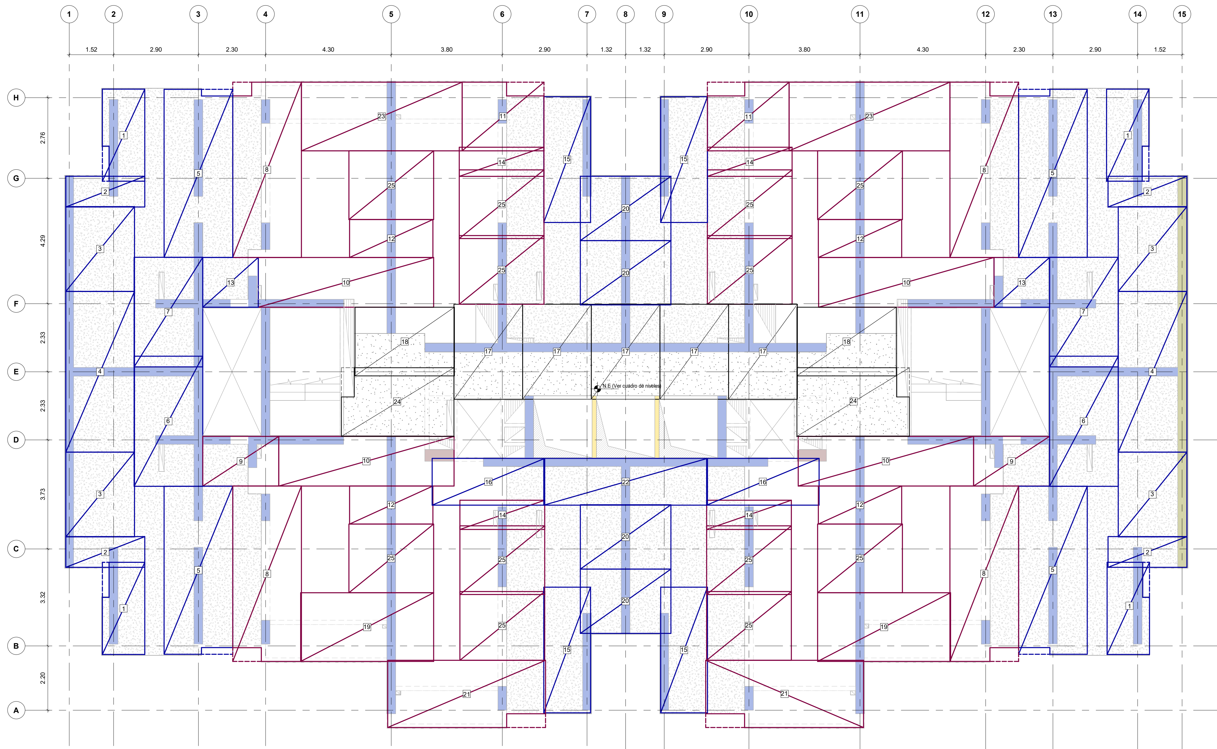
PLANTA DE REFUERZO SUPERIOR PISO TIPO 1 (PISO 3 A PISO 15) Escala 1 : 75
